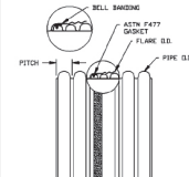
12"-60" (300-1500mm) N-12 WT IB
